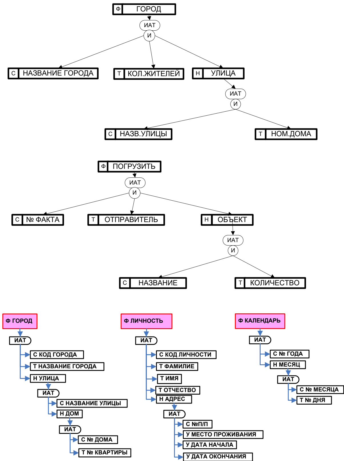
Рис.11. Примеры фреймов
